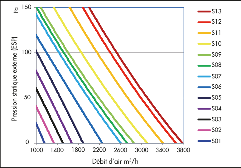
ADG ECO 140PH - courbes de pression statique externe
