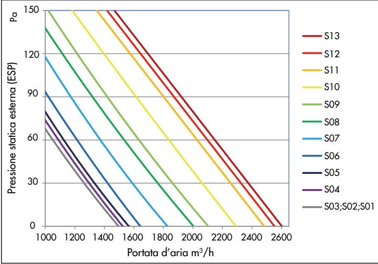
ADG ECO 100PH - curve di pressione statica esterna
