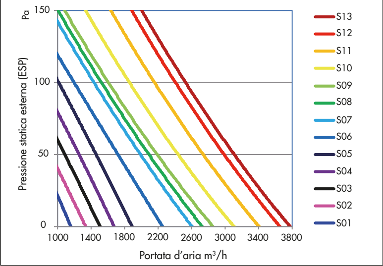
ADG ECO 140PH - curve di pressione statica esterna
